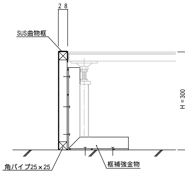
断面図 S = 1 : 5
